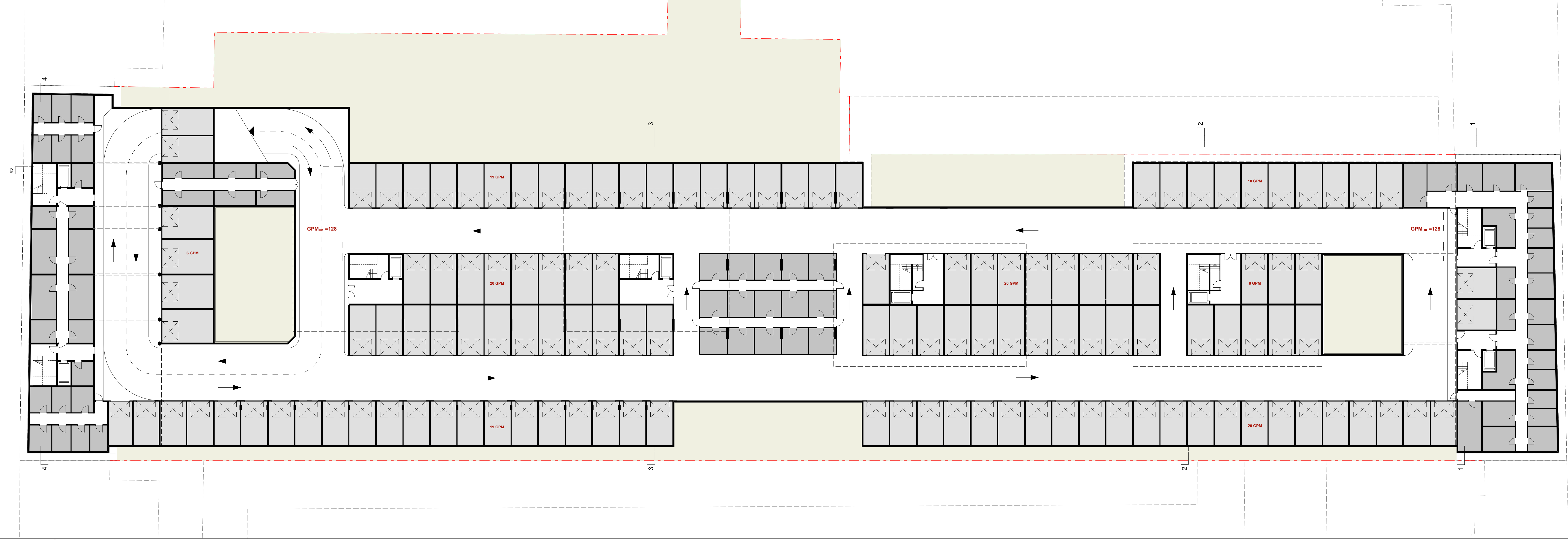
TLOCRT GARAJE -2 M 1:250
