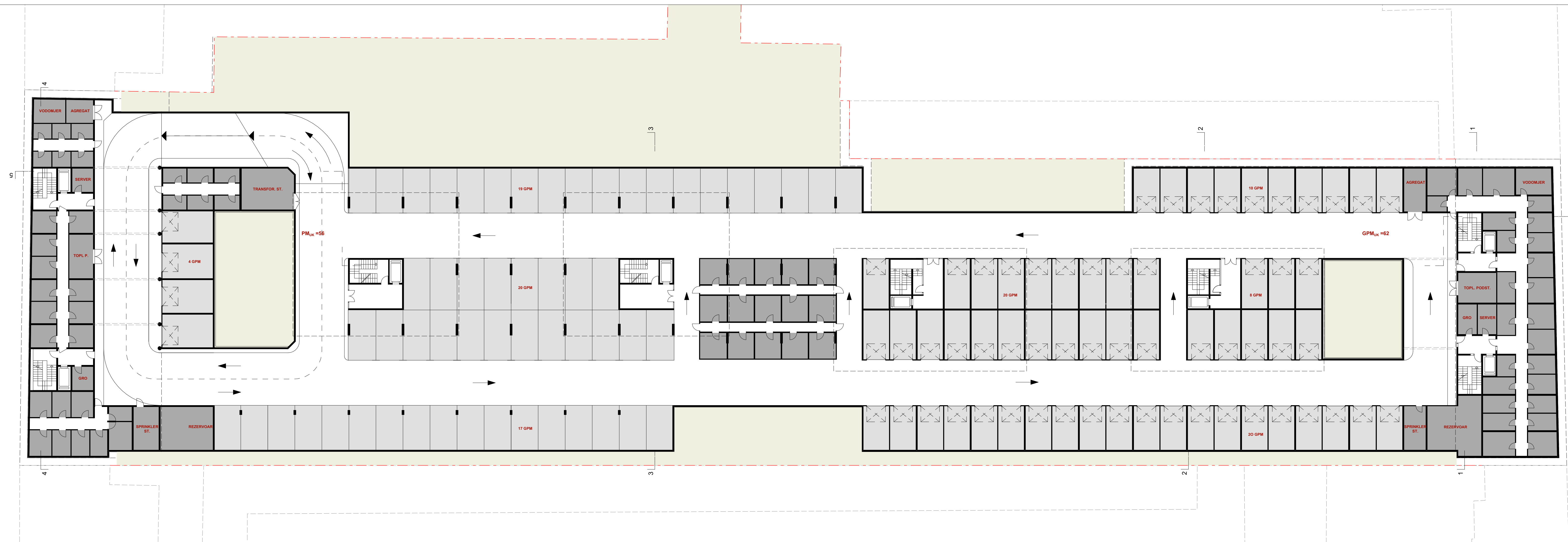
TLOCRT GARAJE -1 M 1:250
